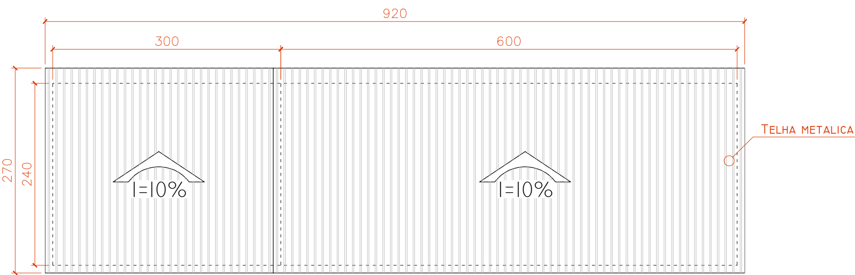
COBERTURA Escala.....1:50
