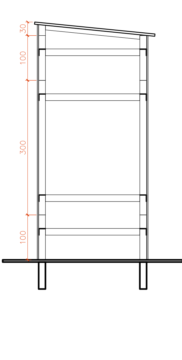
CORTE C Escala.....1:50
