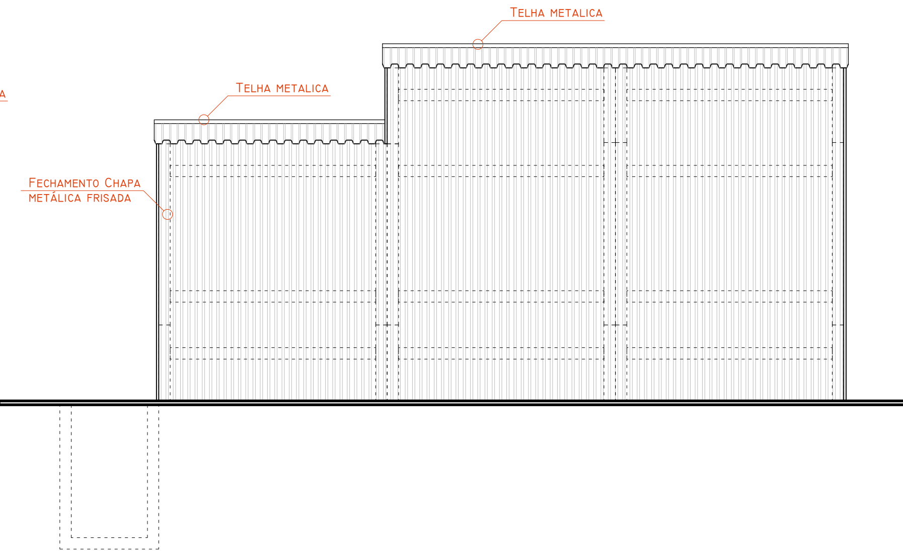
FACHADA 01 Escala.....1:50
