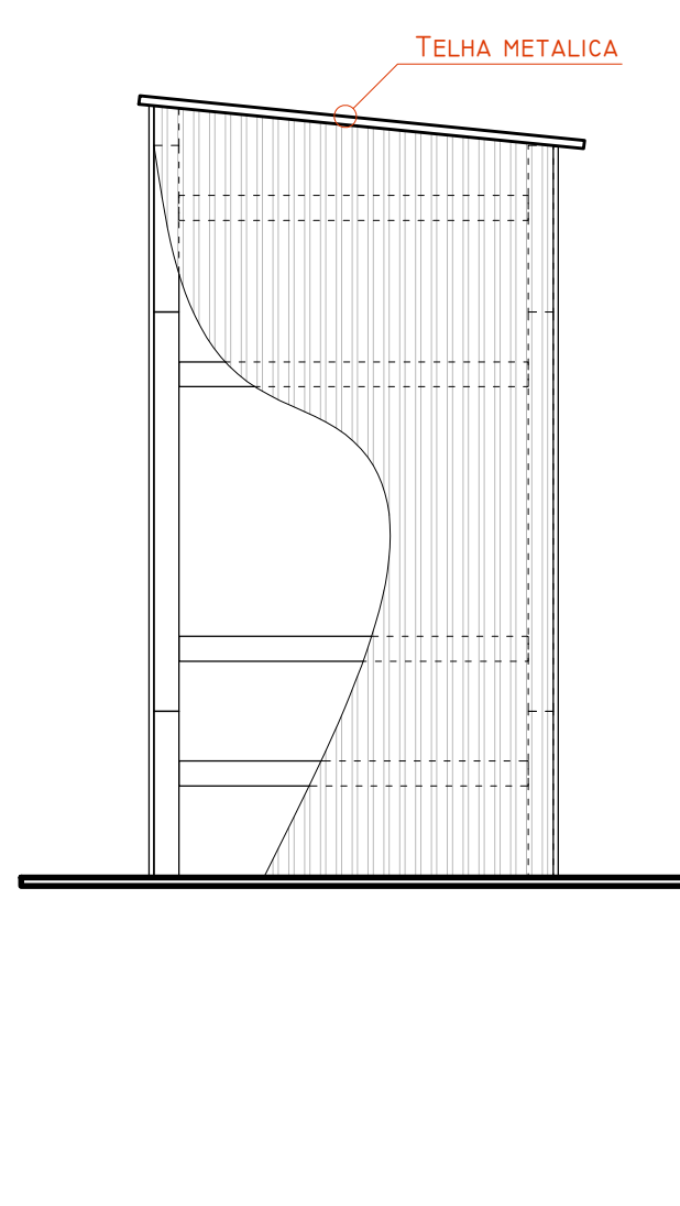
FACHADA 03 Escala.....1:50
