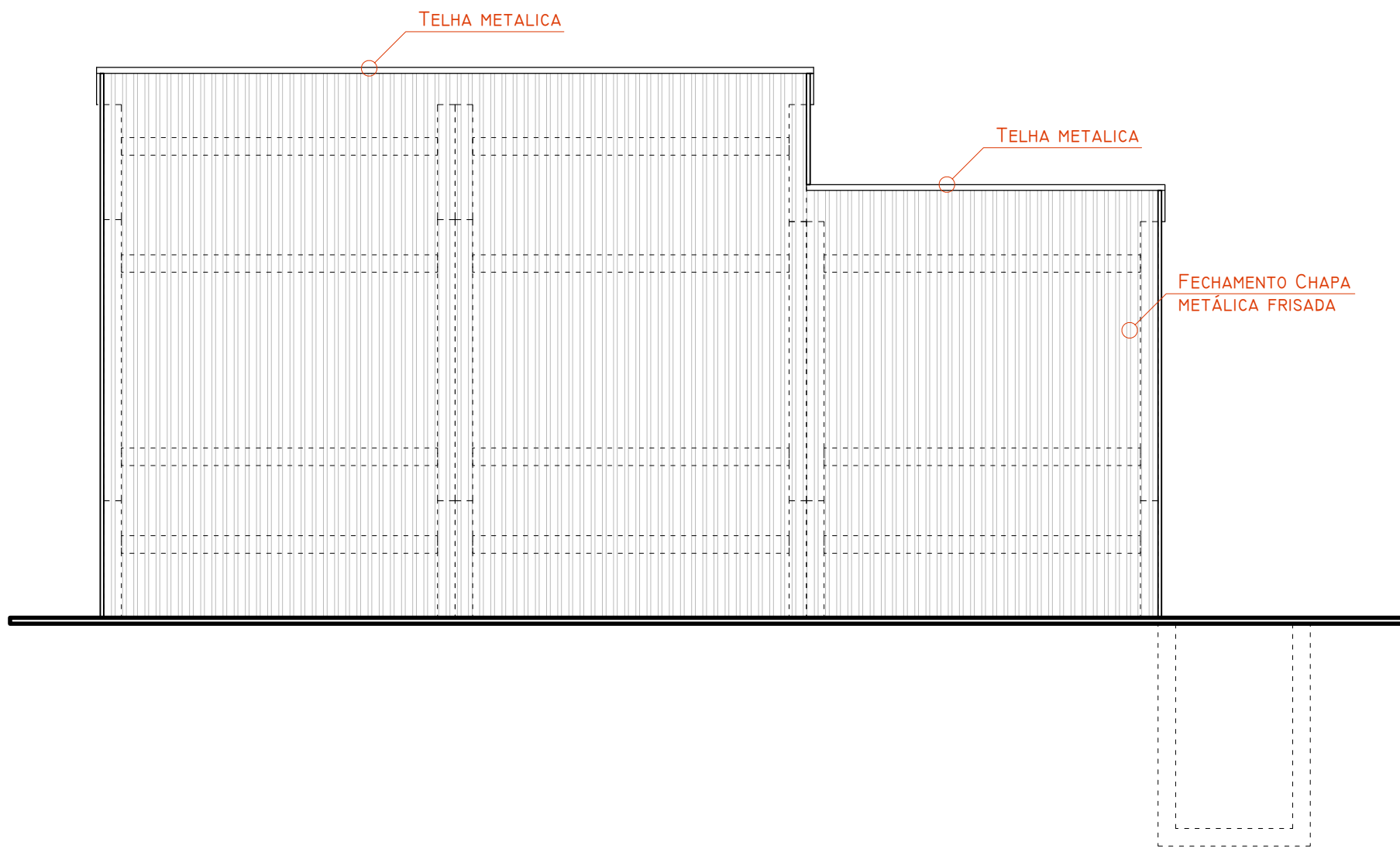
FACHADA 02 Escala.....1:50
