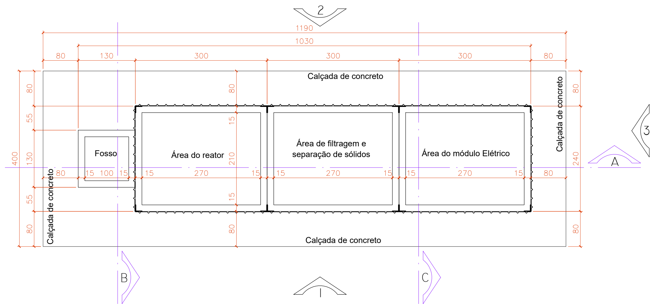
PLANTA BAIXA Escala.....1:50
