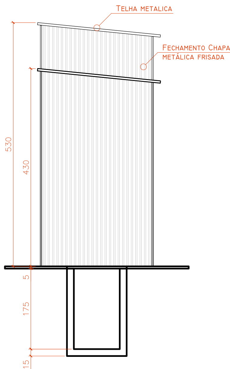
CORTE B Escala.....1:50
