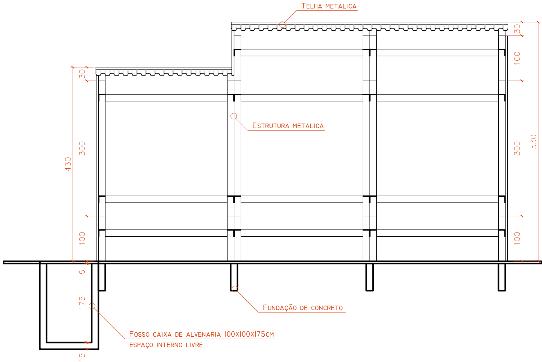
CORTE A Escala.....1:50
